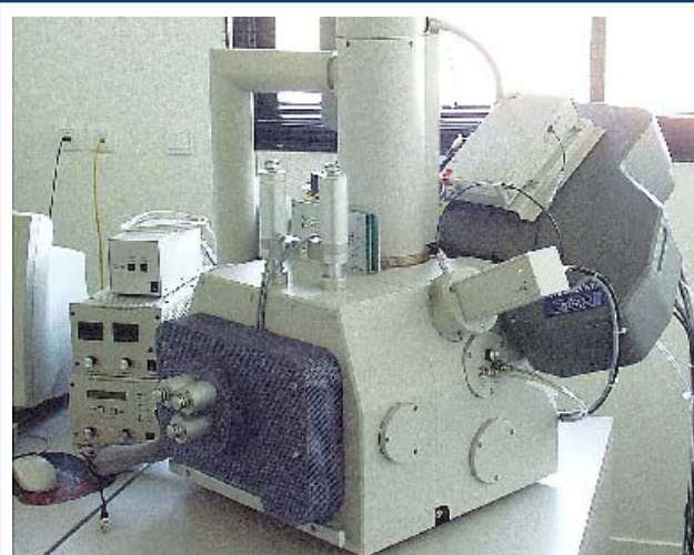
Chambre d'analyse du microscope électronique à balayage (ESEM). Cette chambre de grande dimension (40x40 cm) est équipée de deux systèmes d'analyse X (dispersif en énergie et en longueur d'onde) et d'une platine chauffante atteignant 1500°C. (photo, IRAMAT-CEB/CNRS)
